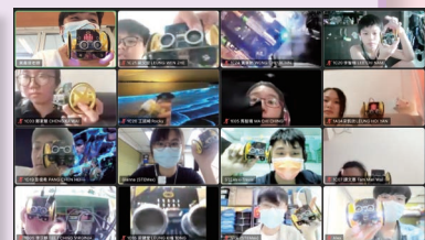
初中學生在家進行「動手動腦」的STEM學習活動。
