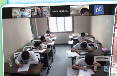
在內地設試場，為跨境生安排公平、公正的呈分試。
